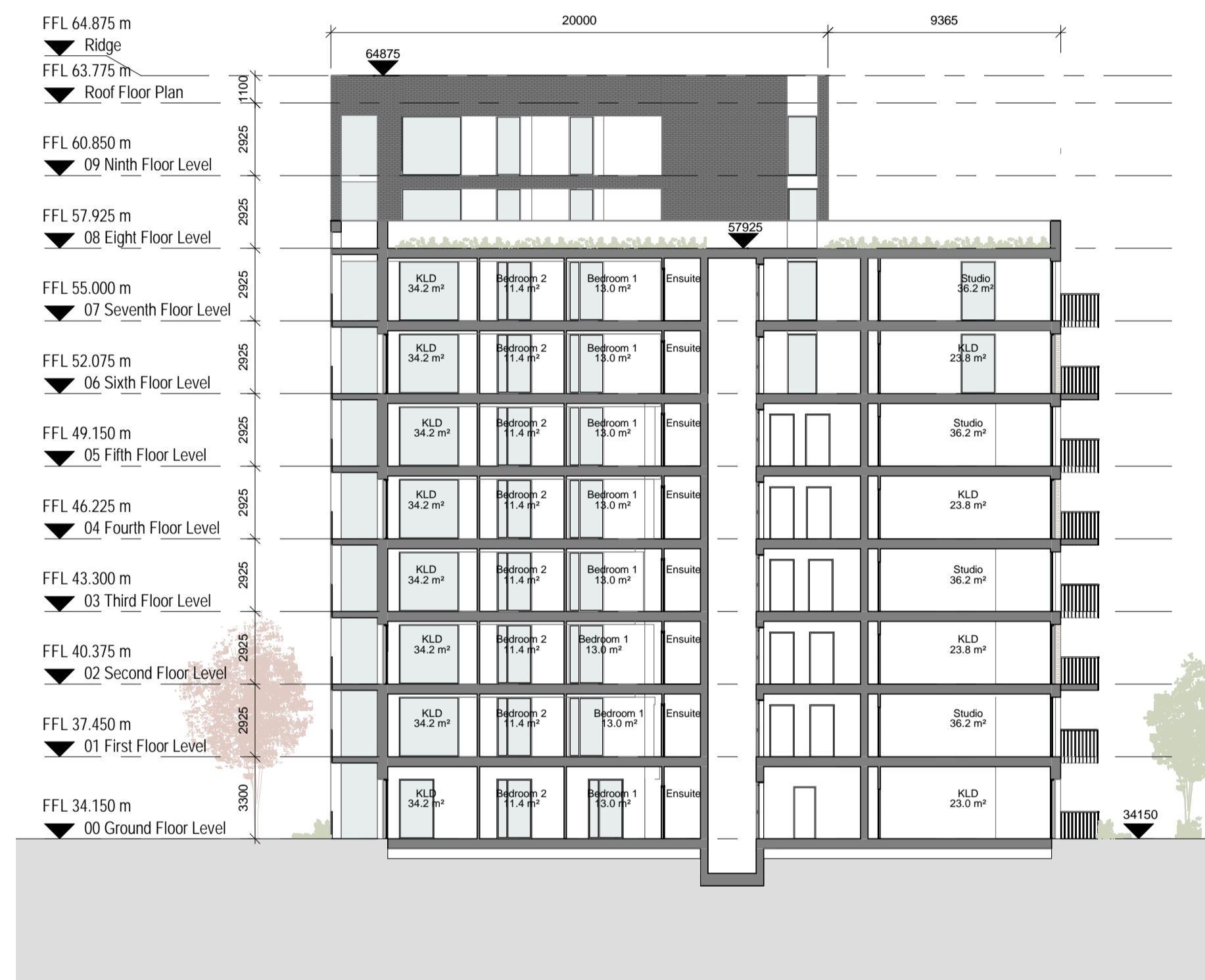
1 Cross Section B 1 : 200
